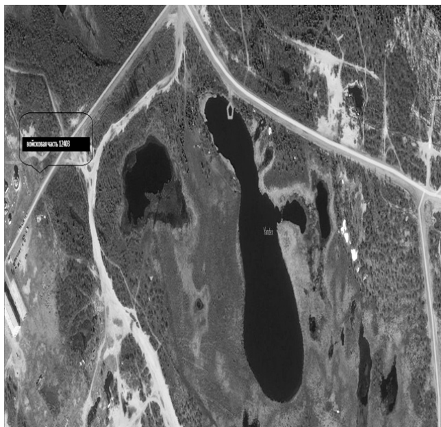
СХЕМА 14 подъезд к естественному источнику противопожарного водоснабжения в р-не полигона ТБО
