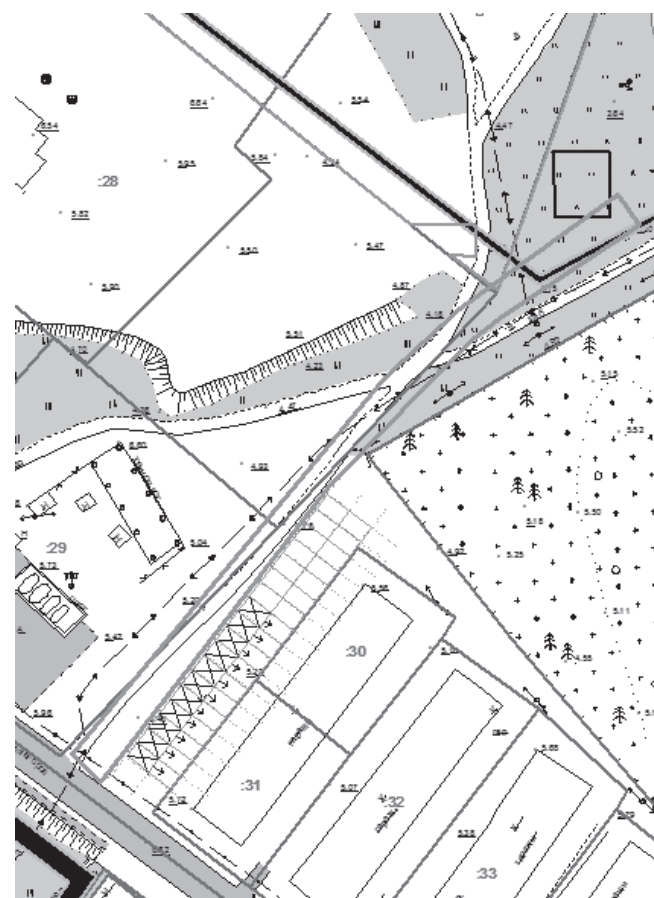
СХЕМА 11 подъезда к естественному источнику противопожарного водоснабжения в районе дома 19Б по ул. Первомайская
